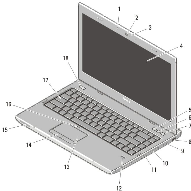
Afbeelding 3. Vostro 3450: vooraanzicht
